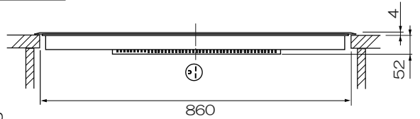
正面図
