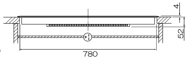
側面図
