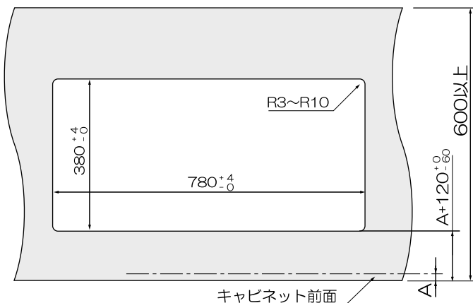
取り付け穴 (ワークトップの開口寸法)
